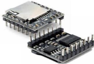
Gambar 4. DF Player Mini
